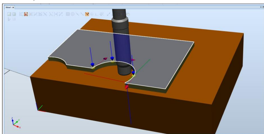
Рис. 15. Задание точек на объекте (продолжение)
