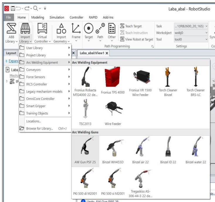
Рис. 9. Добавление сварочной горелки
