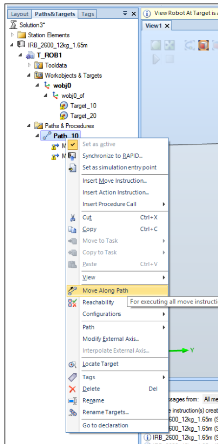
Рис. 20. Перемещение робота вдоль траектории
