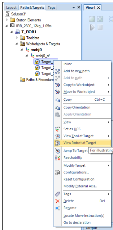
Рис. 16. Перемещение робота в точку
