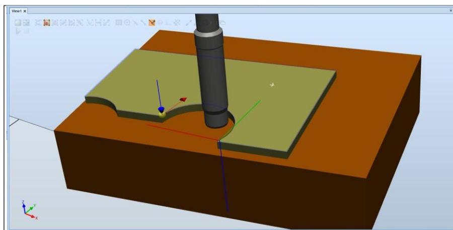
Рис. 14. Задание точек на объекте
