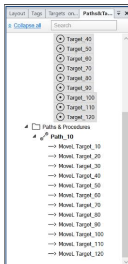
Рис. 18. Перемещение точек в траекторию движения
